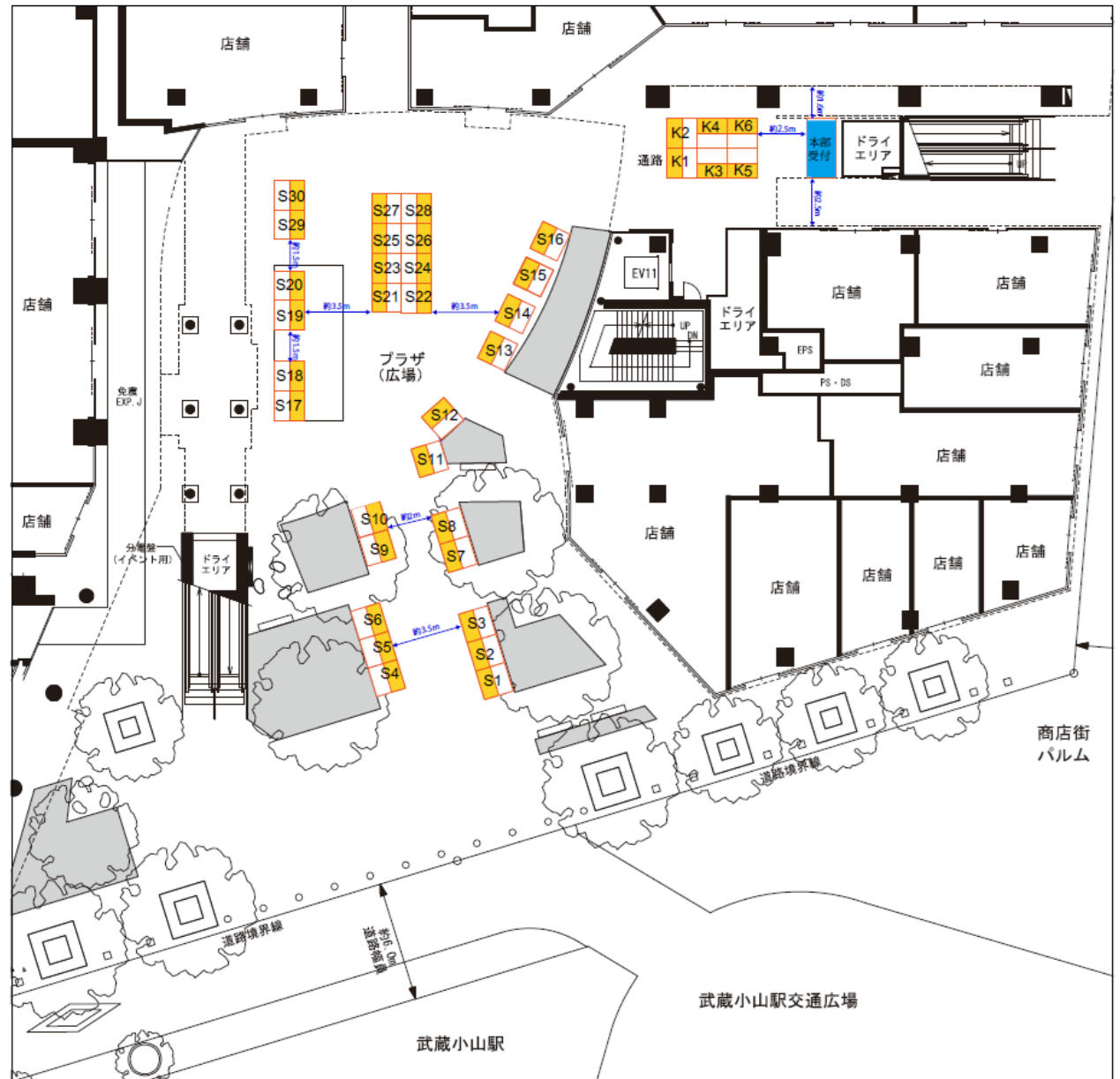
敷地配置図・1階平面図 (1:200)
