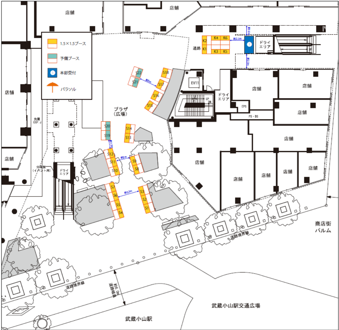
敷地配置図・1階平面図 (1:200)
