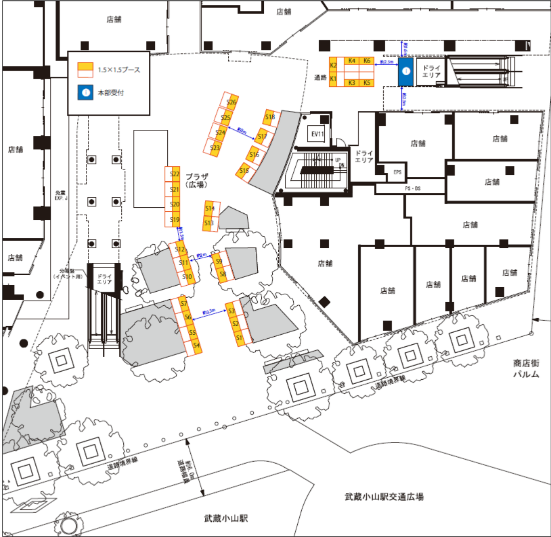
敷地配置図・1階平面図（1：200）
